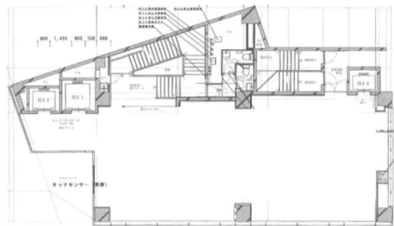
2階平面図
